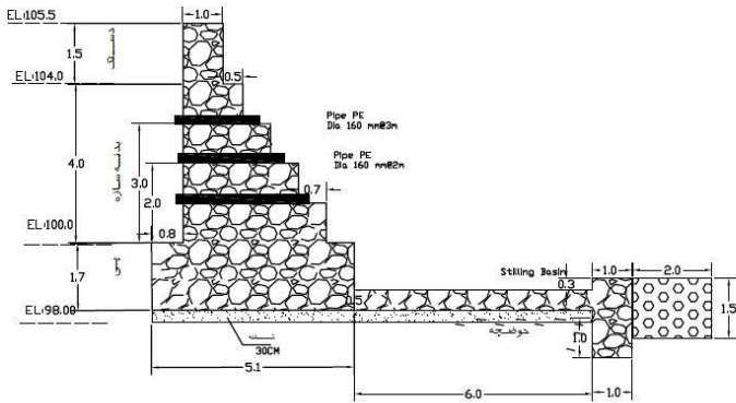
Section A-A ESCALA 1.....100 پلان کلی سازه
