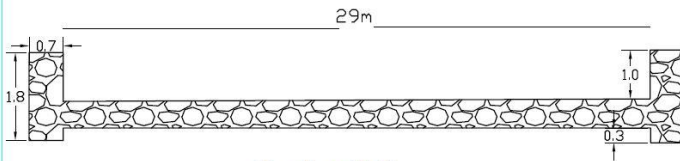
Section C-C ESCALA 1.....100
